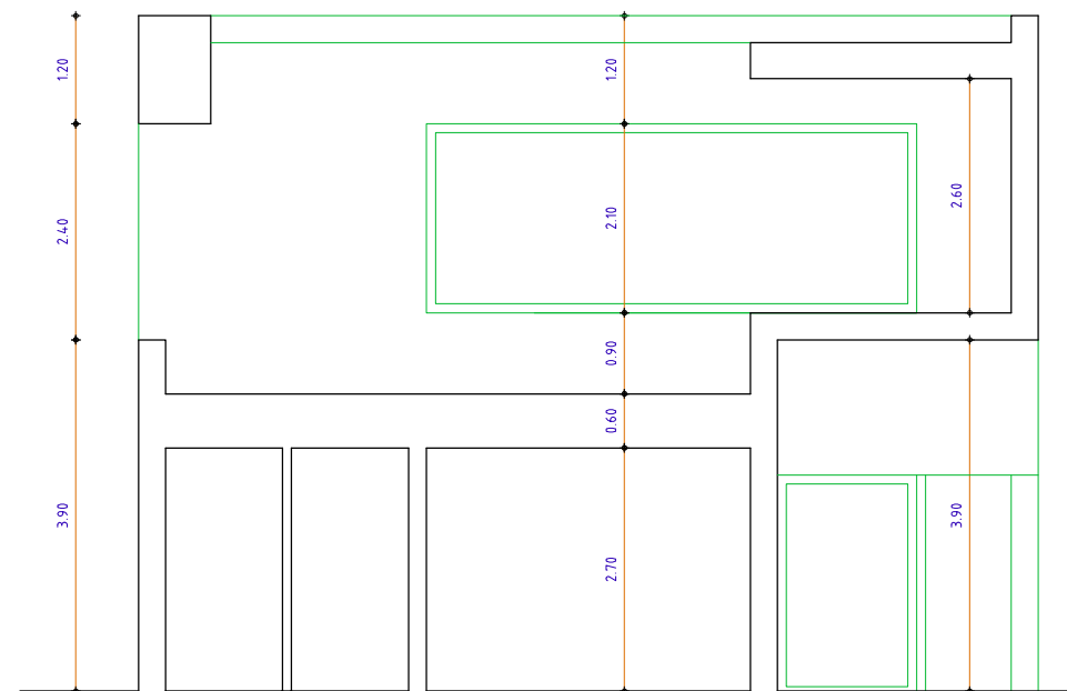
SECCION A-A
